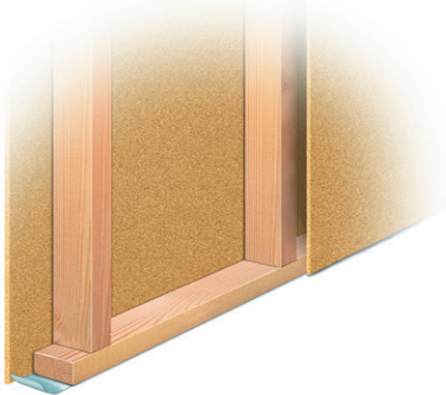
R 15. Vegg med stomme av träreglar min. 45x70 mm, c ≤600 mm, på båda sidor försedd med min. Byggelits 12 mm spånskivor.
