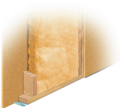
EI 30. Vegg med stomme av träregrar min. 45x70 mm c ≤ 600 mm, på båda sidor försedd med Byggelits 12 mm spånskivor. Mellan reglarna ska finnas min. 70 mm isolering av stenull.
