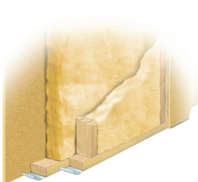
EI 60. Vegg med dubbel träregrarstomme eller korsande reglar min. 45x70 mm c ≤ 600, på båda sidor försedd med Byggelits 12 mm spånskivor. Mellan reglarna ska finnas min. 2x70 mm isolering av stenull.
