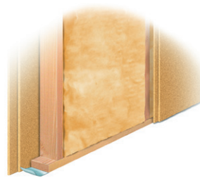
REI 60. Vegg med stomme av träreglar min. 45x120 mm c ≤600 mm, på båda sidor försedd med min. Byggelits 26 mm*) spånskivor. Mellan reglarna ska finnas min. 120 mm isolering av stenull.
