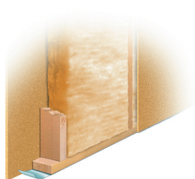
EI 60. Vegg med stomme av träregrar min. 45x95 mm c ≤ 600, på båda sidor försedd med Byggelits 12 mm spånskivor. Mellan reglarna ska finnas min. 95 mm isolering av stenull.
