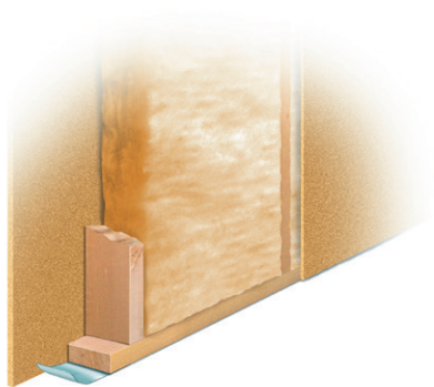
EI 30. Vegg med stomme av träregrar min. 45x95 mm c ≤ 600 mm, på båda sidor försedd med Byggelits 12 mm spånskivor. Mellan reglarna ska finnas min. 95 mm isolering av mineralull.
