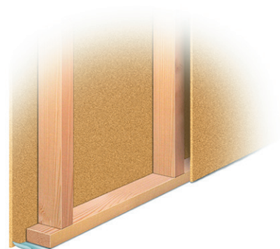
EI 30. Vegg med stomme av träreglar min. 45x70 mm c ≤600 mm, på båda sidor försedd med Byggelits 12 mm spånskivor.
