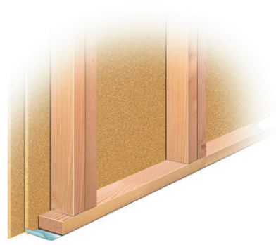
EI 30. Vegg med dubbla träregrar min. 45x70 mm c ≤ 600 mm, på en sida försedd med min. Byggelits 24 mm*) spånskivor.
