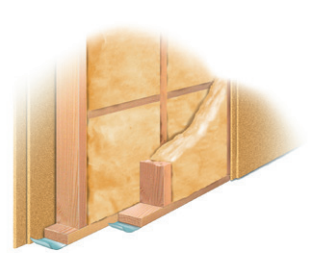
REI 60. Vegg med dubbel träregelstomme, min. 45x120 mm, c ≤600 mm, på båda sidor försedd med min. Byggelits 24 mm*) spånskivor. Träreglarna ska vara avstyvade med kortlingar eller likvärdigt åtminstone på mitten. Mellan reglarna ska finnas min. 2x120 mm isolering av mineralull.
