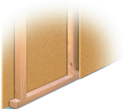
EI 15. Vegg med stomme av träreglar min. 45x45 mm c ≤600 mm, på båda sidor försedd med Byggelits 12 mm spånskivor.
