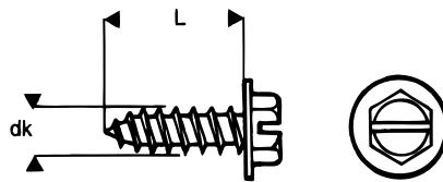
Gjengepresset AB-gjenge med uttrukket spiss. Sekskanthode med meiselspor.
