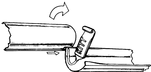
Skjøting med fugemasse (B)
