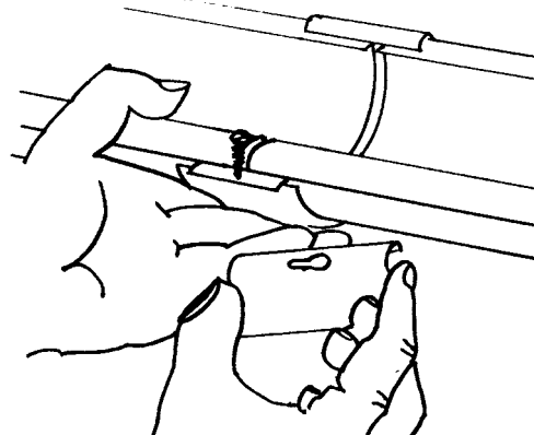
Skjøting med skrueskjøtestykke 40 (C)
