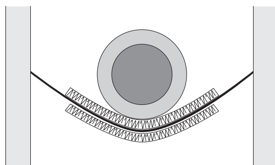
Innebygd kanal. Tilleggisolering av patentband med cellegummi.
