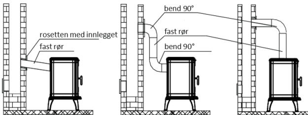
Fig. 3 Skjema for kobling av peisovn.
