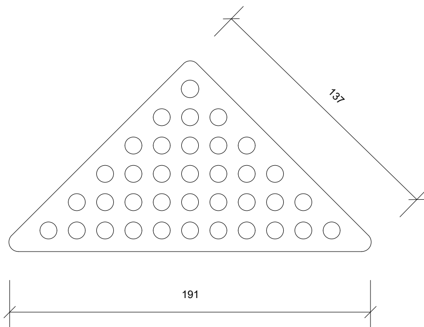
Plan/Plan/Draufsicht
