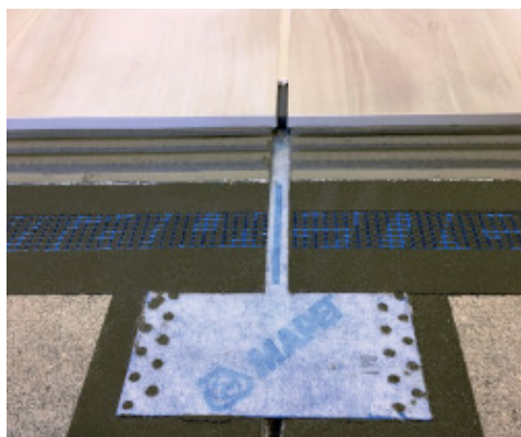
Mapeband Easy lagt over en fleksibel fuge i avrettingslaget
