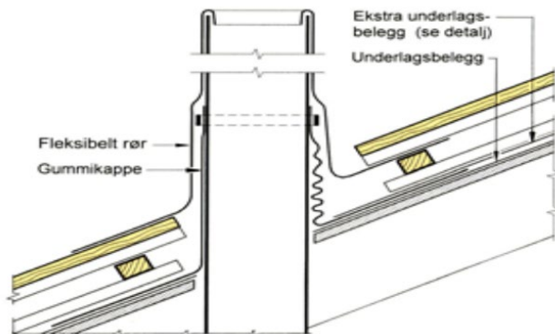
Fig. 66 b Gjennomføring for avtrekk Inntekking av soilrør med gummikappe som tres over og festes mot rør og underlagsbelegg. Kappens flens dekkes med nytt underlagsbelegg. Over soilrør og kappe tres et fleksibelt rør med plate. Røret bøyes over soilens ende. Plata tilpasses over/under tekningsbordene.
