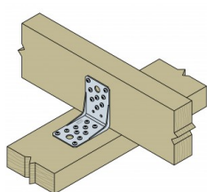
Tre-tre skjøt
