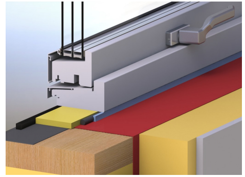
Fig 4. Vinduet skal tettes med diffusjonstett innside, isolasjon, samt vind og vann avvisende utside.
