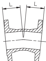
S-9668 Flensebend 22 1/2°
