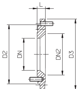
S-9667 Reduksjonsflens med varmfor-sinkede pinner skruer
