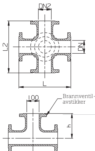
S-9663 Flensekryss Med brannventilavstikker
