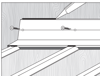
7 Skru profilen i veggen. Fug på overkanten av toppinndekningen og på underkanten ned mot dekklisten.
