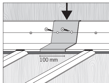
9 Skjær 100 mm av toppinndekningen og bruk det som overlapp over skjøten på toppinndekningen.
