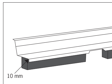
6 Monter ekspanderende fugebånd under toppinndekningen, 10 mm fra kanten.
