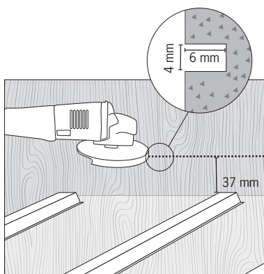
5 Fres en fuge i veggen 37 mm over dekklistene. Skjer fugen i en høyde på min. 4 mm og i en dybde på min. 6 mm.
