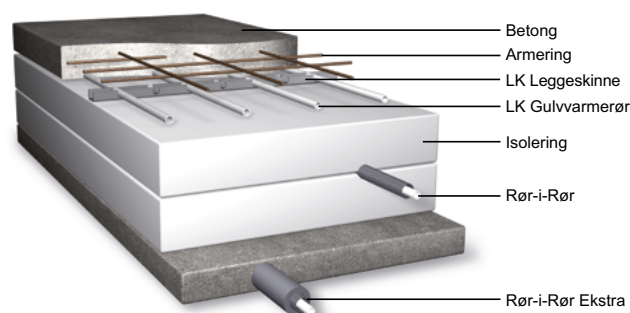
Forlegging av Rør-i-Rør i betongplate med gulvvarme.
