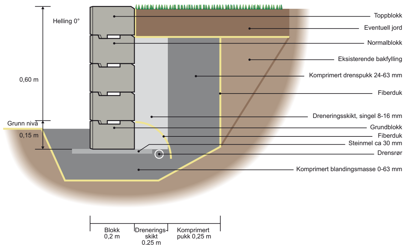
Bilde 1. Seksjonstegning for mur opp til 0,6 m.
