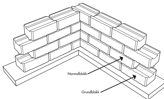
Bilde 9. Innvendig 90° hjørne.
