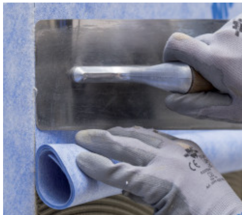
Montering av neste lag
