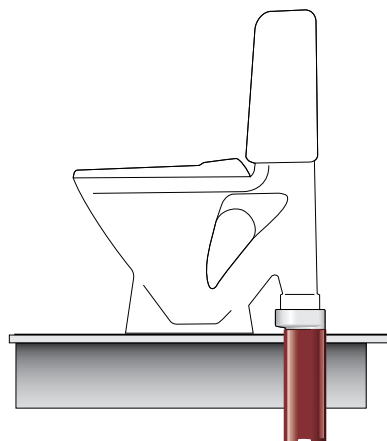
Fig. 5. Tilkobling av klosett med S-lås. Benytt KJ-MA® Rør og en av KJ-MA SYSTEM® klosettilkoblinger.
