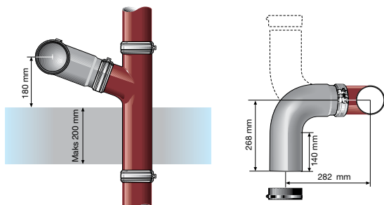
Fig. 1. Tilkobling av ett eller to klosetter med P-lås til side for vertikal samleledning med etasjegrør 70° og enkelt eller dobbelt klosettband 90°.
