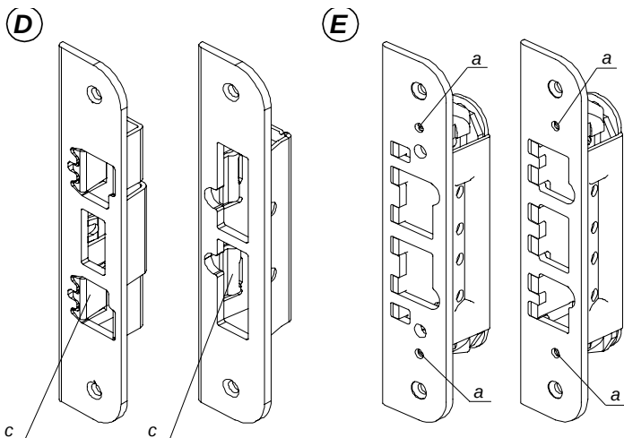
Figur D. Mekanisk justering, ved bøying av metalltungen "c".
