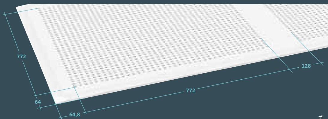
Montering. Forsenket kort- og langkant
