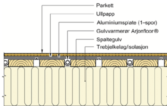
Figur: Spaltegulv
