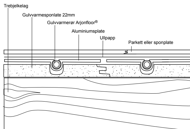
Figur: Sponplater med spor for gulvvarme
