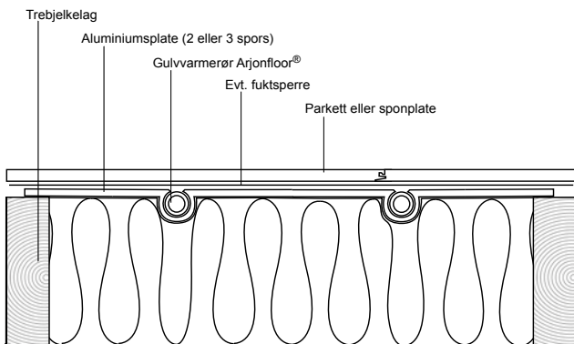
Figur: Trebjelkelag
