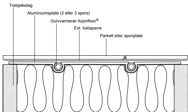
Figur: Trebjelkelag
