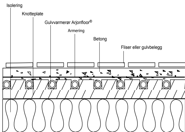
(Det kreves min.200mm isolasjon inklusive knotteplate og min.30mm betong over varmerør) ill6 Figur: Knotteplate
