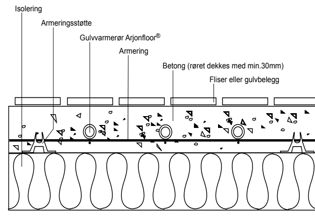
Figur: Strips til armering
