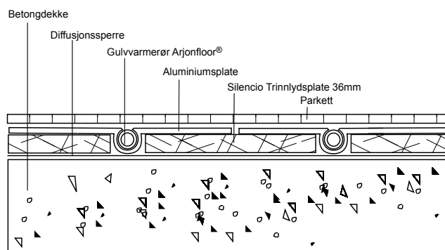
Figur: Silencio Thermo
