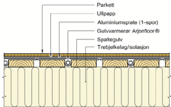
Figur: Spaltegulv
