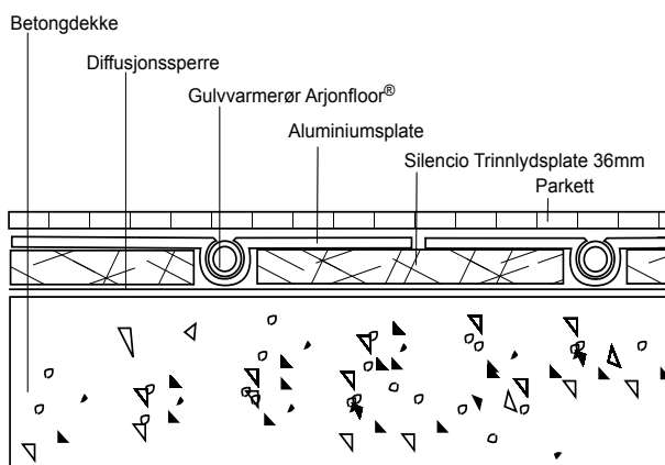
Figur: Trinnlydplater på betong-/hulldekke
