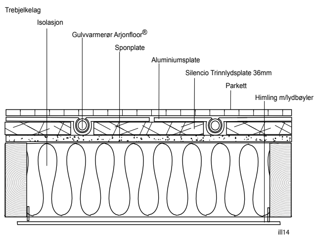
Figur: Trinnlydplate på trebjelkelag
