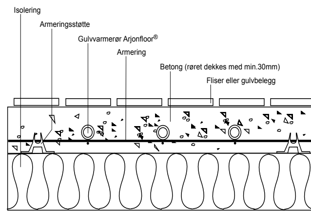
(Det kreves min.200mm isolasjon og min.30mm betong over varmerør) ill7 Figur: Strips til armering
