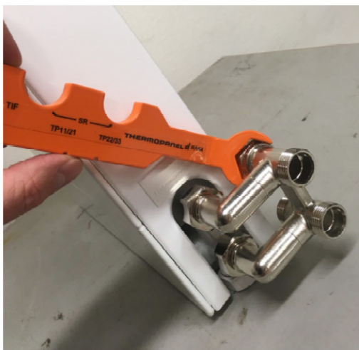
Demontering av ventilinsats
