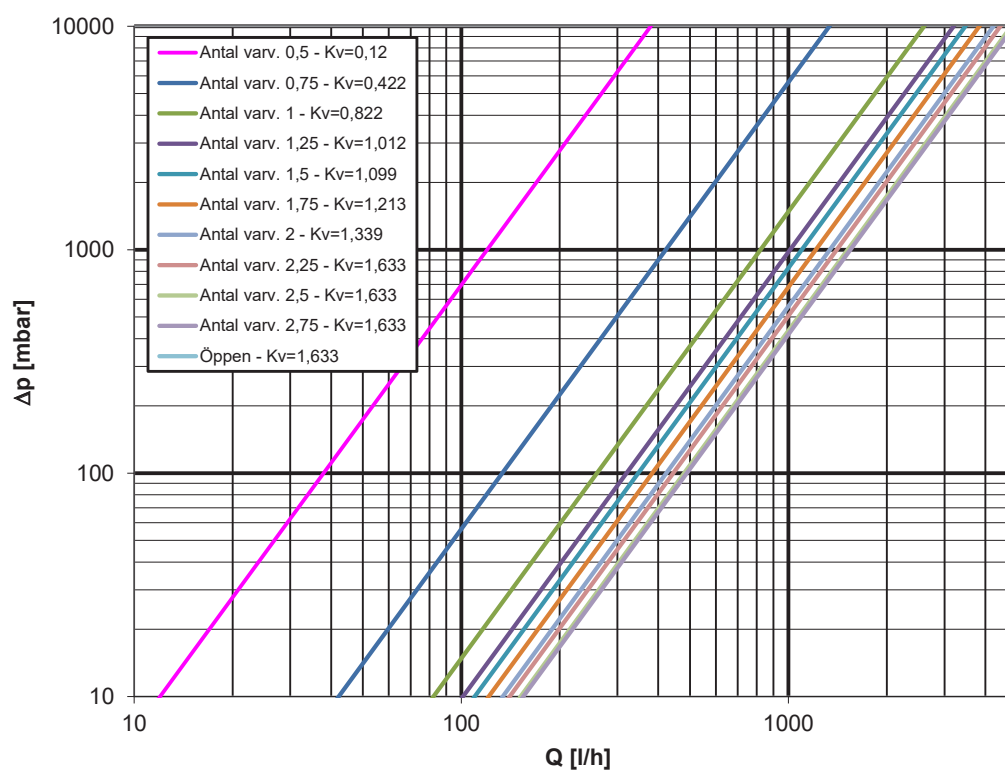
Tryckfallsdiagram RAK4
