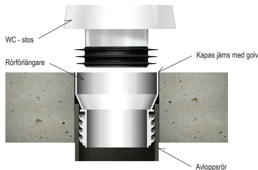
A Rörförlängare Excentrisk 10 mm RSK 310 67 12 NRF 619 66 75
