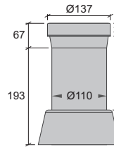
B + K3 WC - Stos 4", Centrisk RSK 310 67 24
