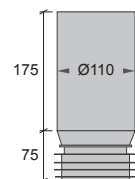
A Rörförlängare Centrisk RSK 310 67 07
