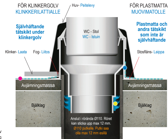
A Rörförlängare Centrisk RSK 310 67 07
