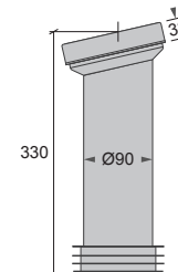
A + K3 WC - Stos, Vinklad RSK 310 67 23
