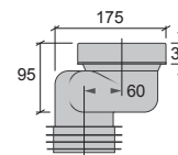
A + K2 WC - Stos Offset 60, Excentrisk 60 mm RSK 310 66 78 NRF 619 66 53
