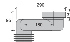
A + K2 WC - Stos Offset 180 Excentrisk 180 mm RSK 310 66 81 NRF 619 66 56
