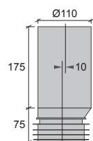
A Rörförlängare Excentrisk 10 mm RSK 310 67 12 NRF 619 66 75
