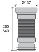
A WC - Stos, Flexibel RSK 310 66 98 NRF 619 66 52
