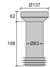
D + K3 WC - Stos 90, Centrisk RSK 291 03 92 NRF 619 66 58
