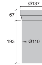
C + K3 WC - Stos 110 muff Centrisk RSK 310 66 86
