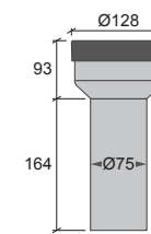
E + K3 WC - Stos 75, Centrisk RSK 310 67 22
