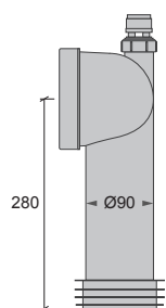
A + K3 WC - Stos, Universal X-tra, Vakuumentil RSK 310 66 61V
