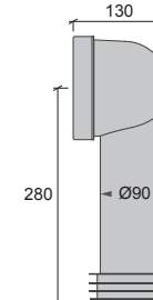
A + K3 WC - Stos, Universal RSK 310 67 20 NRF 619 66 71
