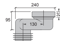
A + K2 WC - Stos Offset 130 Excentrisk 130 mm RSK 310 66 80 NRF 619 66 55
