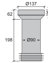
A + K3 WC - Stos 110, Centrisk RSK 310 66 85 NRF 619 66 57
