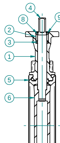
DN 125/200
