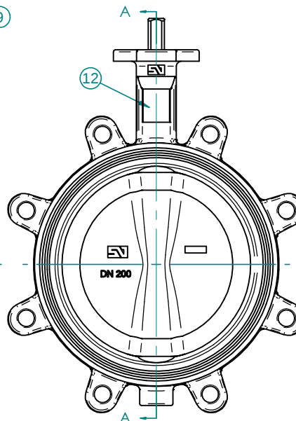
DN 125/200
