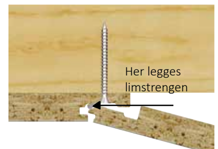
Fig. 2 Låseprofil
