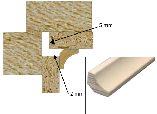
Fig. 4 Innvendig hulkilist
