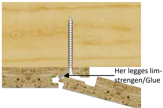
Fig. 2 Låseprofil/Locking profile
