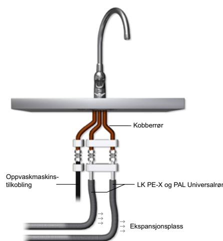
Akseptabel løsning ved installasjon av kjøkkenarmatur med tilkoblingsrør av kobber med LK PE-X og PAL Universalrør RiR.
