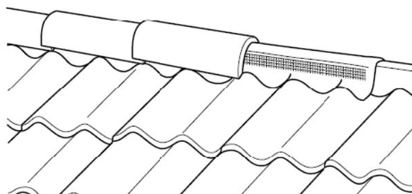
Snittegning mønestein til Zandaprofil:
