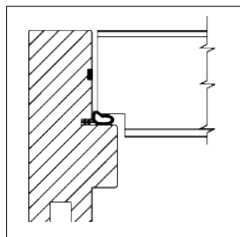
Profil av B-30/35dB dør 52 mm
