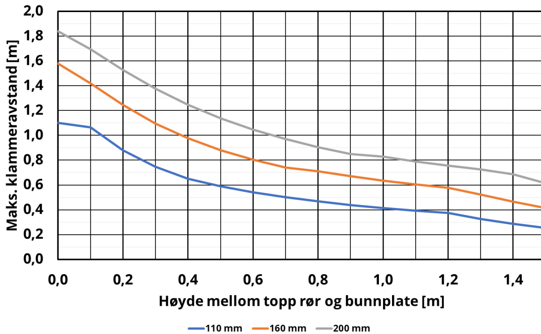
Maksimum klammeravstand i forhold til overdekning for PP SN 8 avløpsrør i skumglass
