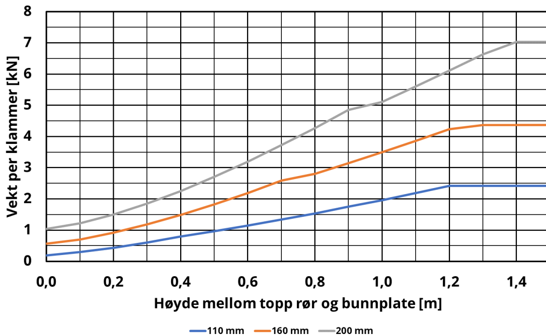
Vekt per klammer i forhold til overdekning og klammeravstand fra diagrammet foran for PP SN 8 avløpsrør i skumglass
