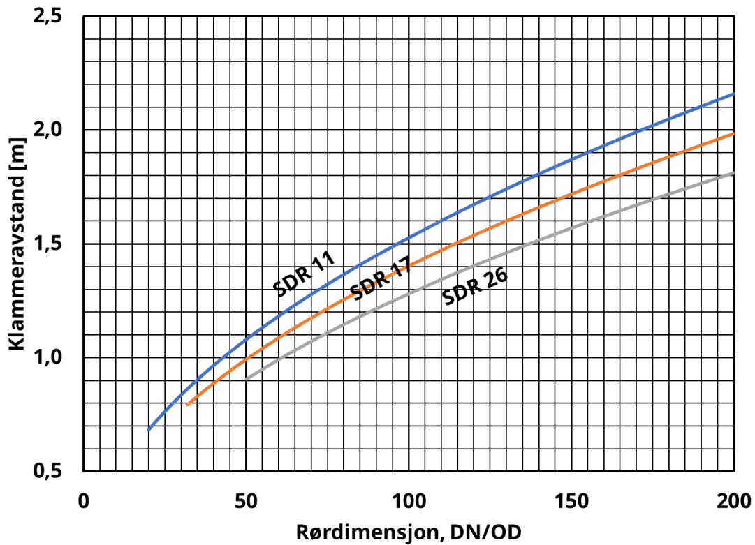
Klamringsavstand horisontale, væskefylte PE 100 trykrør opp til 200 mm med maksimum 10 mm nedbøyning
