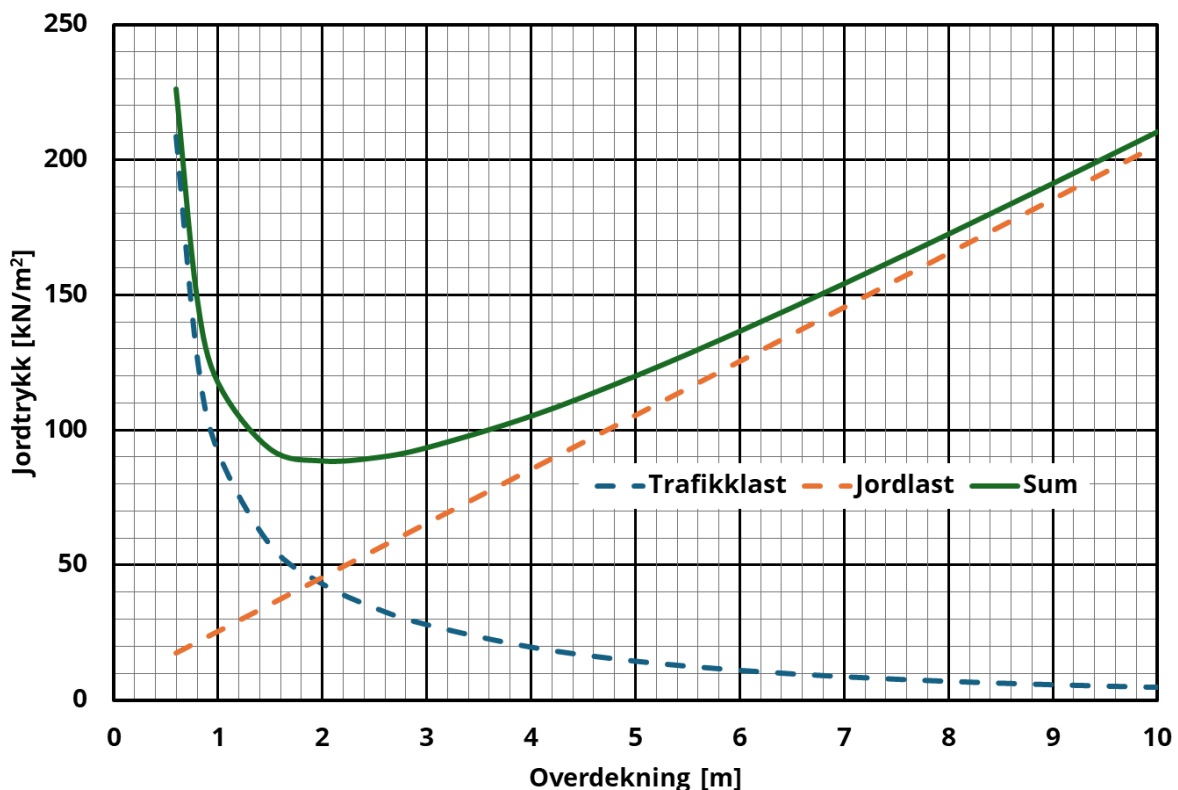
Dimensjonerende laster i offentlig vei (Bk10)
