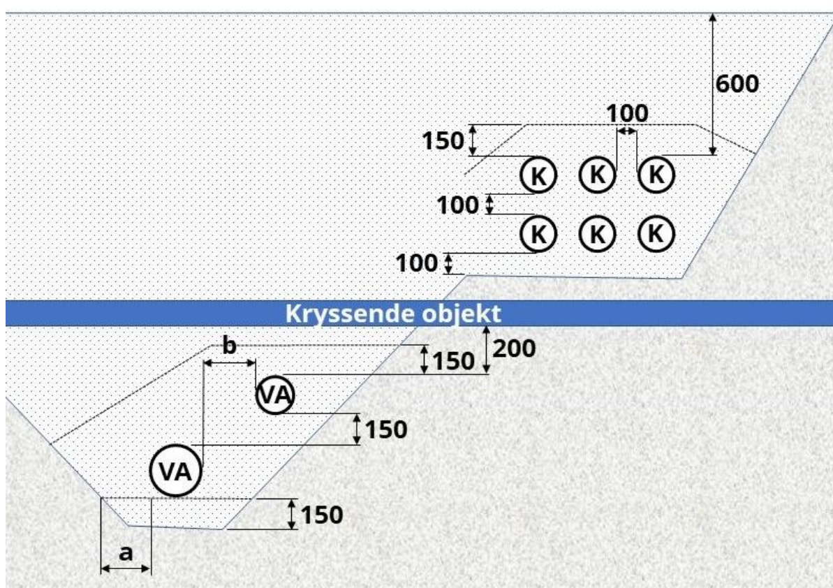
Normale minimumskrav til avstander for vann-, avløps- og drenerør (VA) og kabelvernrør (K) fra leggeanvisningene og NS 3070-1:2015.
