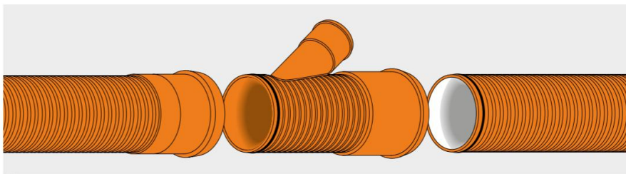
Pragma mufte-ende • Pragma rørdel • Pragma spissende Kontroller og rengjør mufte, gummiring og spissende. Påfør glidemiddel på innsiden av muffen. Skjøt sammen rørene for hånd eller med hjelpemiddel.
