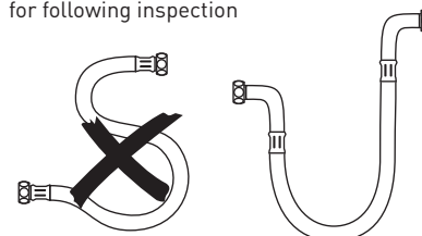
Slangen må ikke få et S-formet bøj Anslutningsslangen får inte monterats som ett S The hose may not get a S-shaped bend
