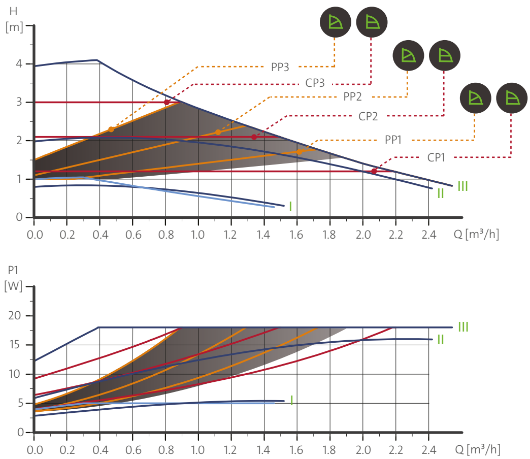
Fig. 37 ALPHA2 og ALPHA3, XX-40
