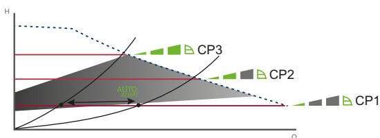
Fig. 26 Tre konstanttrykkurver og -indstillinger
