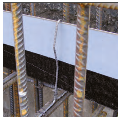
Montering med monteringsklemme på armeringen.
