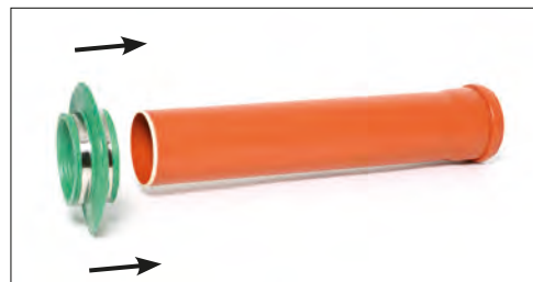
Murkragen skyves på
