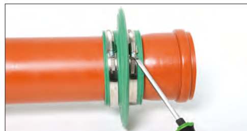
Festes ved at man trekker til strammebåndene
