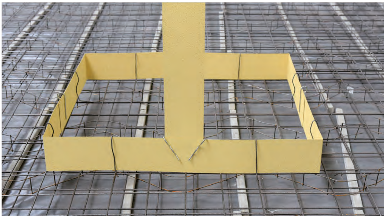
Tetningsplate MB før støpingen. 3 cm innfugingsdybde i betong er tilstrekkelig for trykktett tetting.
