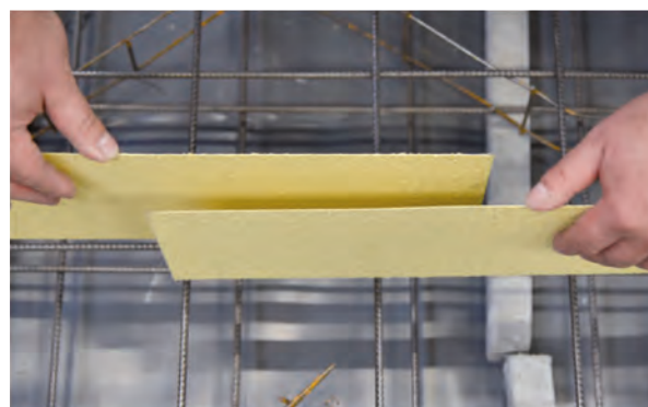
Overlapping i skjøteområdet 20 cm. Ikke nødvendig med klebeskjøt.
