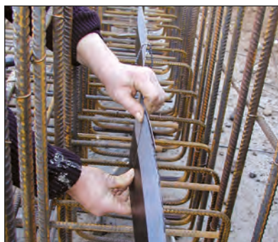
Overlapping og sikring med skjøteklemmer.
