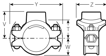
INVÄNDIGT GÄNGAT AVSTICK
