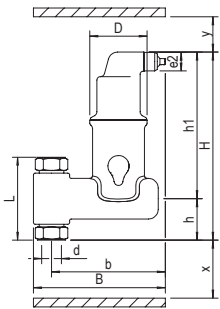
SPIROVENT SOLAR VERTIKAL
