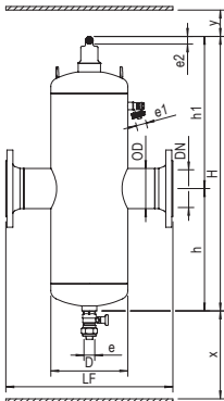
SPIROCOMBI HI-FLOW FLENSSET UTFØRELSE
