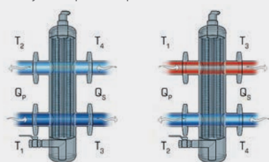
Kjøling
