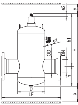
SPIROVENT FLENSSET UTFØRELSE
