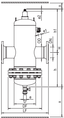
SPIROCOMBI DEMONTERBAR HI-FLOW FLENSSET UTFØRELSE
