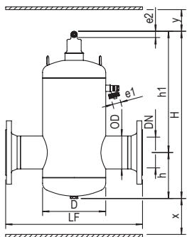
SPIROVENT FLENSSET UTFØRELSE
