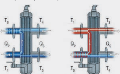
Kjøling
