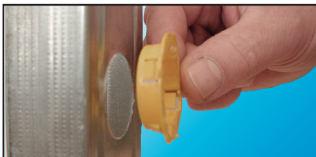
Lag et 35mm hull med f.eks. en hullstanse. Sett inn plastforing.
