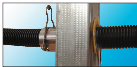
Skyv spikeravviseren mot plastforing, samtidig som røret trekkes i motsatt retning. Monter fikseringsklammer som vist.
