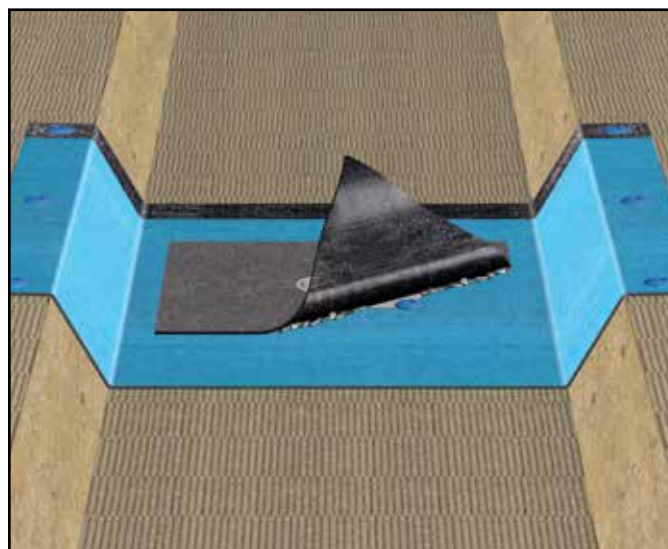
Sluket festes mekanisk, og belegget på sluket helsevises så til Base Syntan. Det er viktig at varmen tilføres undersiden på slukbelegget og ikke direkte på syntan.
