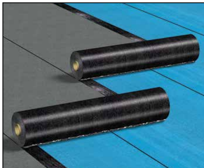
Toppbelegget helsevises til underlaget. Ved bruk av Base Syntan er det viktig å påføre varmen på undersiden av overlagsbelegget, og ikke på den blå syntan-overflaten. Vi anbefaler å skjøte i flak.
