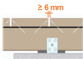
Kantskruing på Kebony Character gir pen terrasse uten synlige festmidler.
