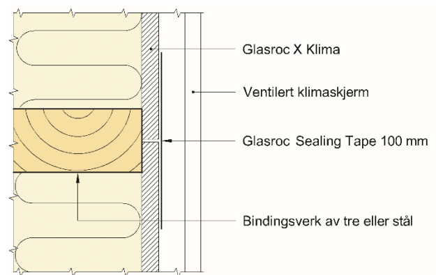
Fig. 3 Horizontal skjøt med understøttelse med 100 mm Glasroc Sealing Tape monterert sentrisk over skjøten.
