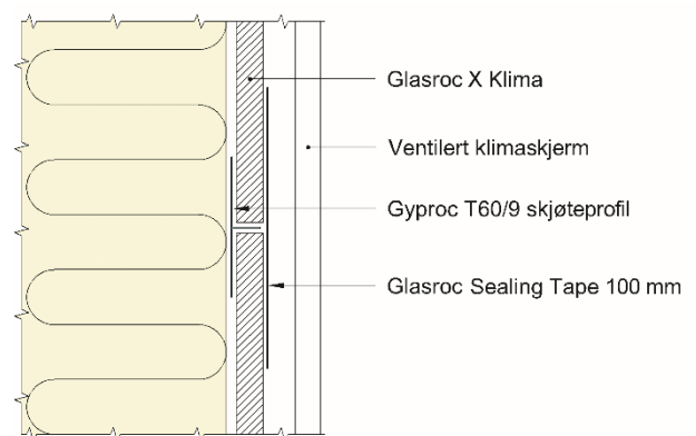
Fig. 4 Horizontal skjøt uten understøttelse med 100 mm Glasroc Sealing Tape monterert sentrisk over skjøten.
