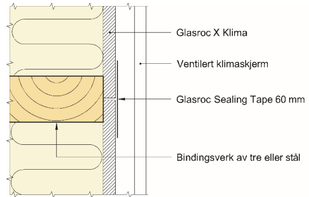
Fig. 2 Vertikal skjøt med Glasroc Sealing Tape 60 mm monterert sentrisk over skjøten.
