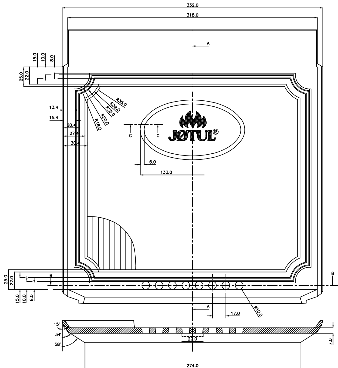
Snitt B-B
