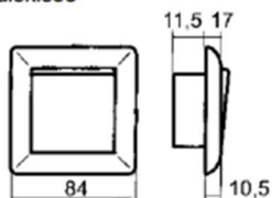
Målskisse
